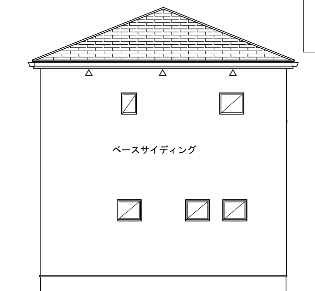
北側立面図 S : 1/100
